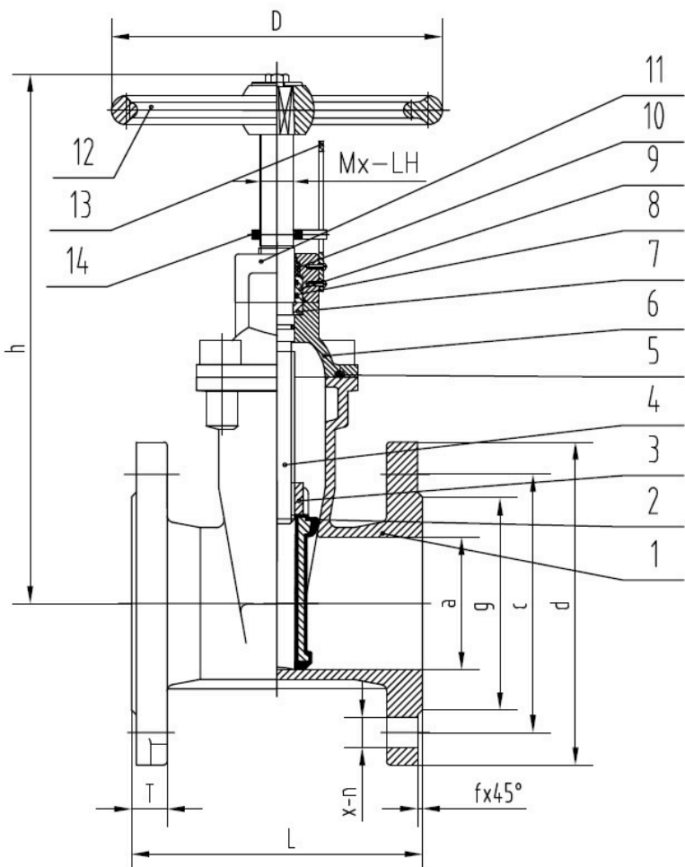
Чертеж габаритный задвижки клиновой чугунной с обрезиненным клином и невыеданным штоком ABRA-A-4-10(16)GiXXX (размеры в таблице ниже):
