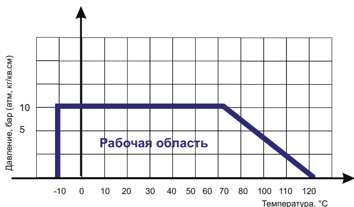
Диаграмма Давление / Температура для задвижки клиновой АВРА-А40-10-XXXG с обрезиненным клином и невыедным штоком Ду 300-900, Ру 10
