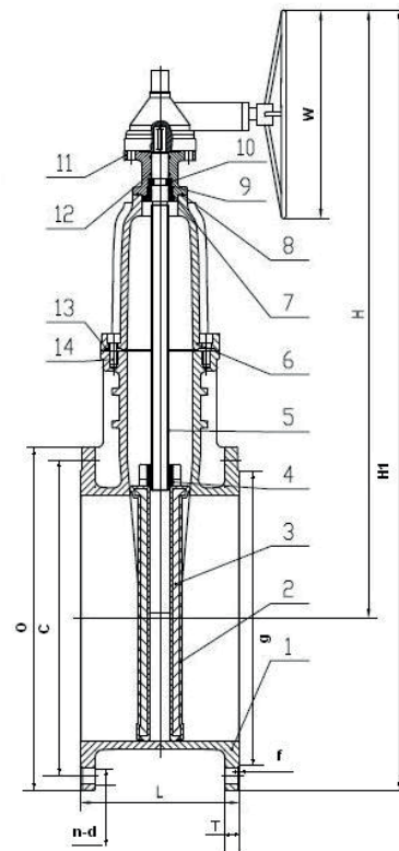
Чертеж габаритный задвижки клиновой с обрезиненным клином и невыдвижным штоком ABRA-A40-10XXXG Ду300-600 чугунной (размеры в таблице ниже, чертеж Ду700-900 еще ниже):
