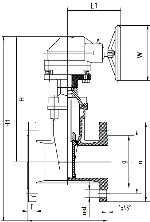
Чертеж габаритный задвижки клиновой с обрезиненным клином и невыдвижным штоком ABRA-A40-10XXXG Ду200-300 чугунной (размеры в таблице ниже, Ду700-900 еще ниже):
